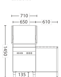
Lato/Side
