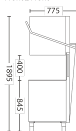
Fronte/Front
