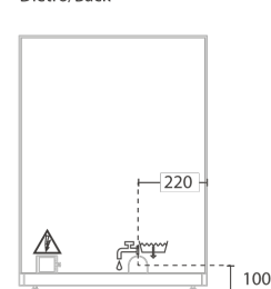
Dietro/Back
