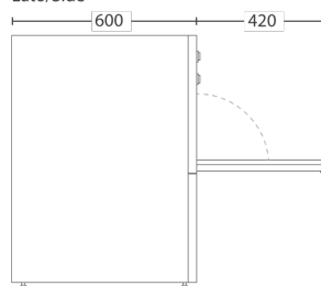
Lato/Side
