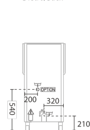
Dietro/Back
